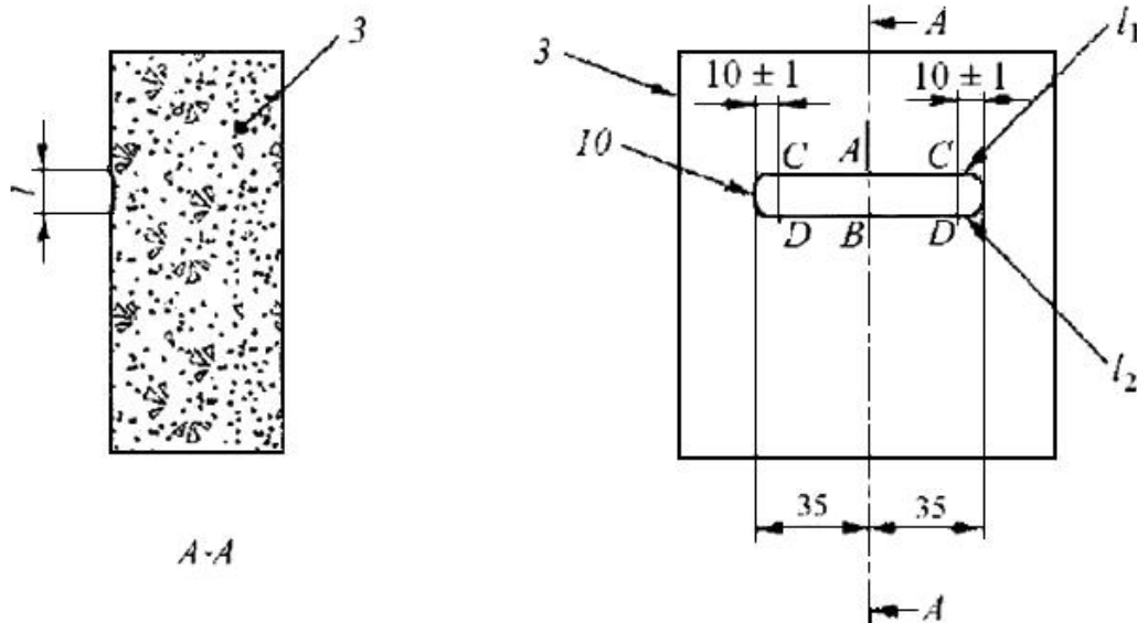
Рисунок В.4 - Схема измерения канавки
